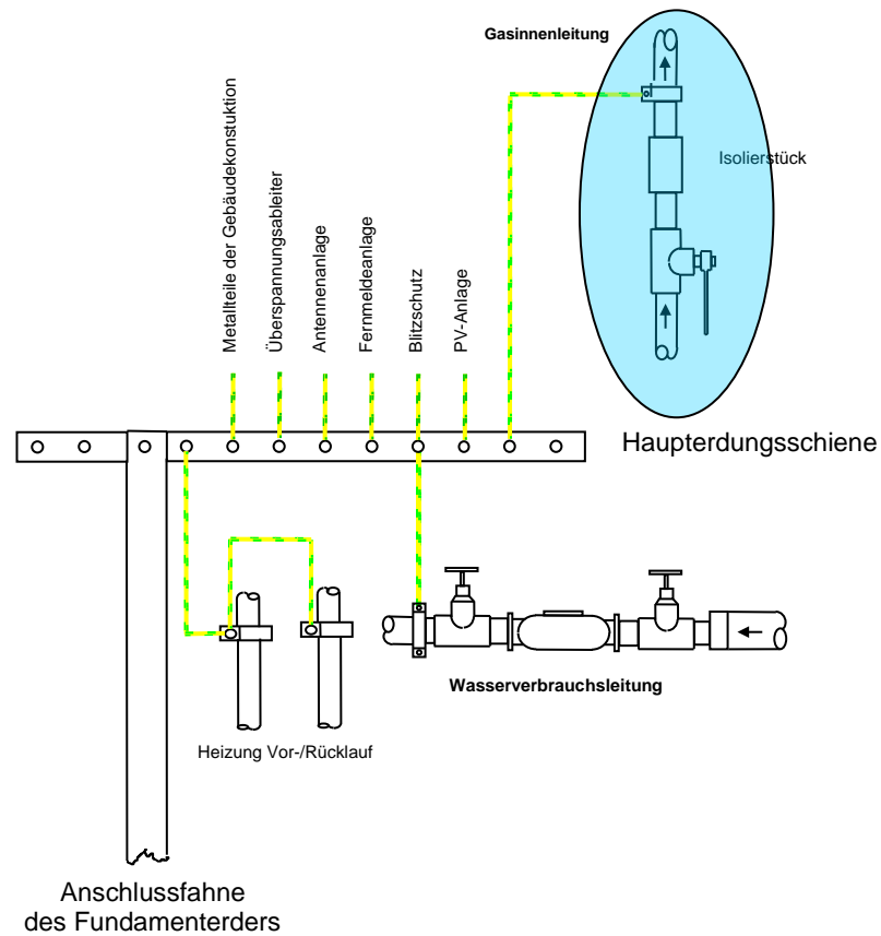
Abbildung 8.4: Schemadarstellung (Schutzpotentialausgleich)
